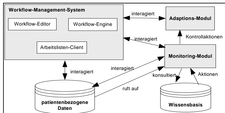
Abb. 1: AdaptFlow-Architektur.
